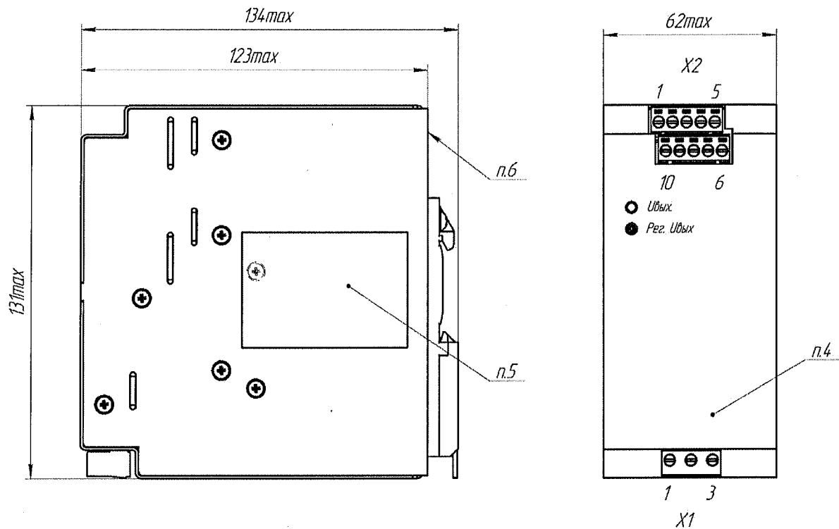
Рисунок Е.6 — Габаритные размеры модуля КАН-Д480
