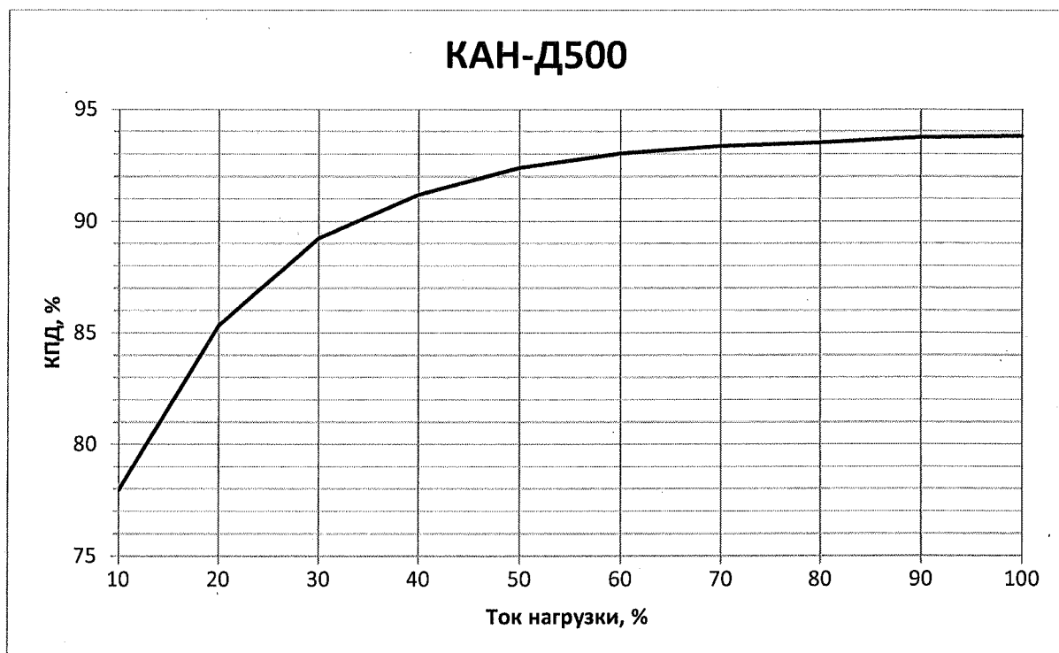
Рисунок Г.20 — График зависимости коэффициента полезного действия от выходной мощности модулей КАН-Д500
