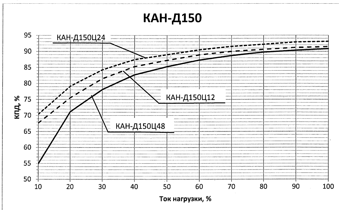
Рисунок Г.16 — График зависимости коэффициента полезного действия от выходной мощности модулей КАН-Д150
