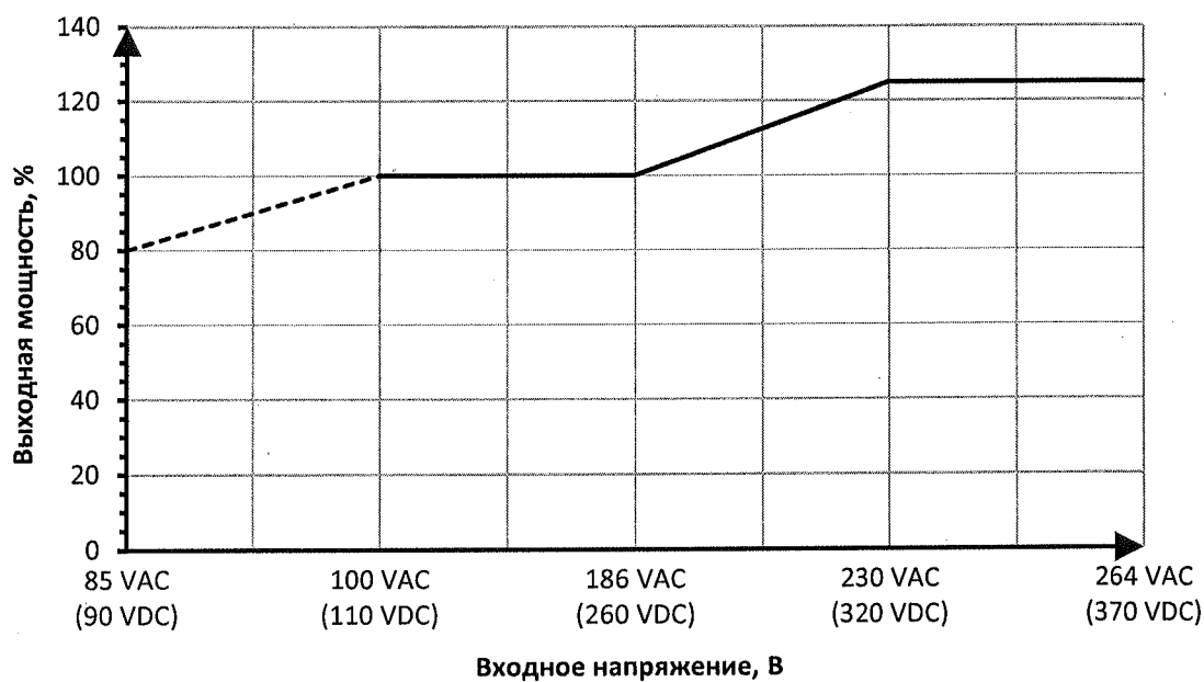
Рисунок Г.11 — График зависимости выходной мощности от входного напряжения для модулей КАН-Д240
