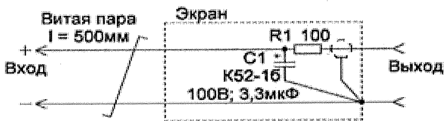
Рисунок 8 — Приспособление для измерения пульсации выходного напряжения
