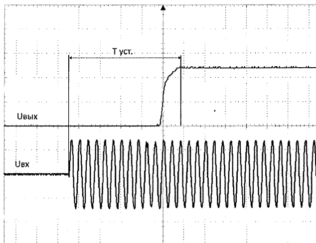
Рисунок 3 – Время установления выходного напряжения
