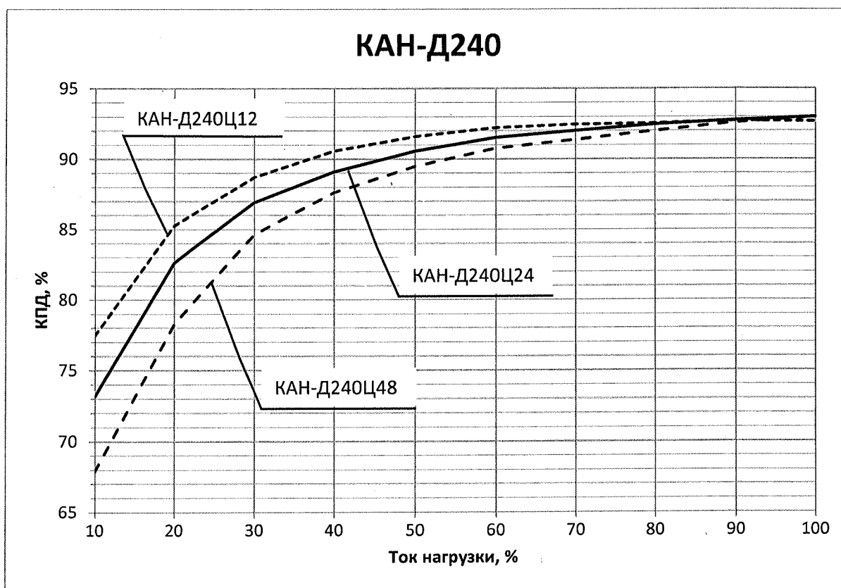
Рисунок Г.17 — График зависимости коэффициента полезного действия от выходной мощности модулей КАН-Д240
