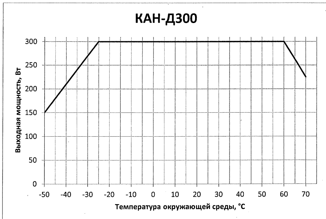
Рисунок Г.5 — График зависимости выходной мощности модуля от температуры окружающей среды для модулей КАН-Д300
