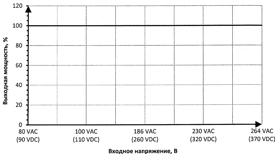
Рисунок Г.10 — График зависимости выходной мощности от входного напряжения для модулей КАН-Д150 и КАН-Д300
